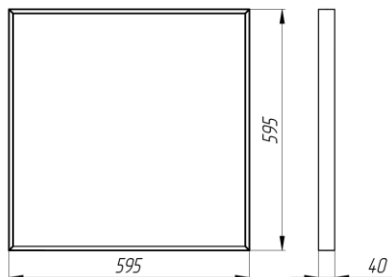
Рисунок 2 — Габаритные размеры светильников серии Офис 595x595x40.
