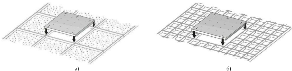
Рисунок 8 — Установка светильника Geniled серии Офис, ЛПО в подвесной потолок.
